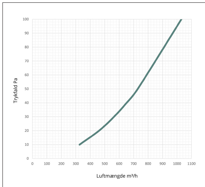
Kapacitetskurve Model A, K-faktor 103
