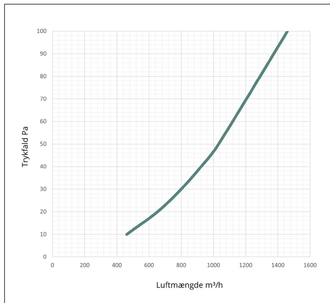
Kapacitetskurve Model B, K-faktor 146
